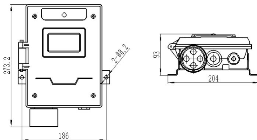
Рисунок 5.1 Габариты
