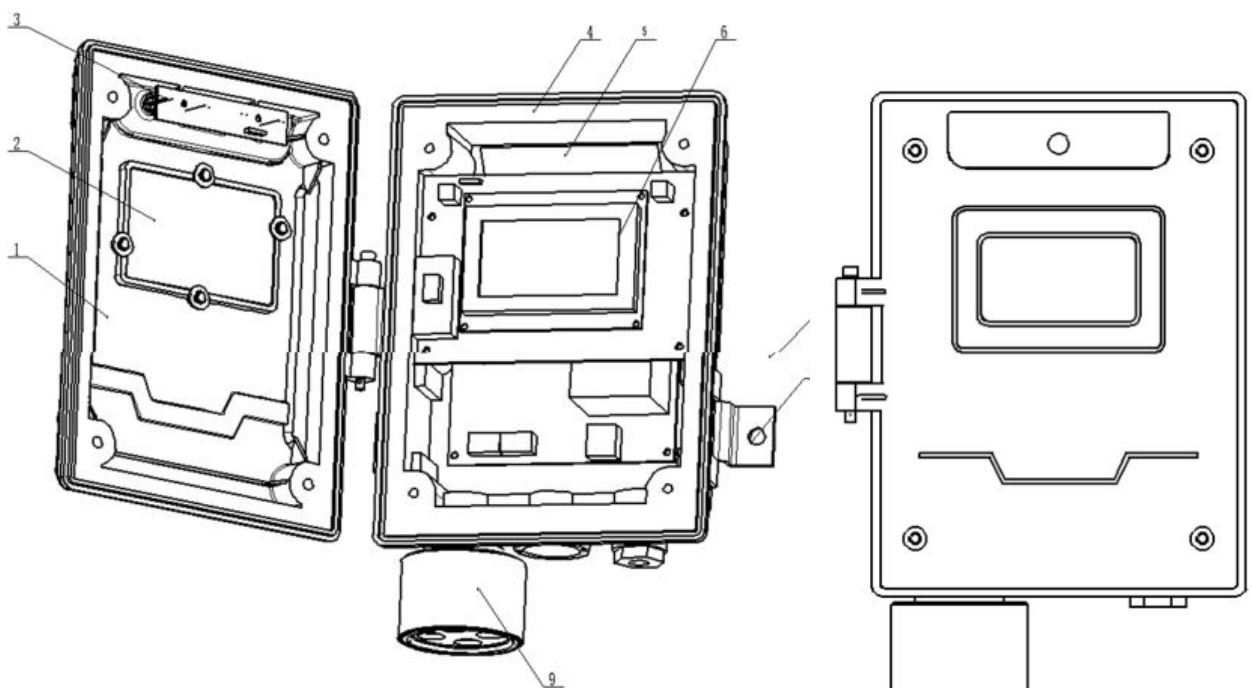
Рисунок 4.1. Внешний вид
