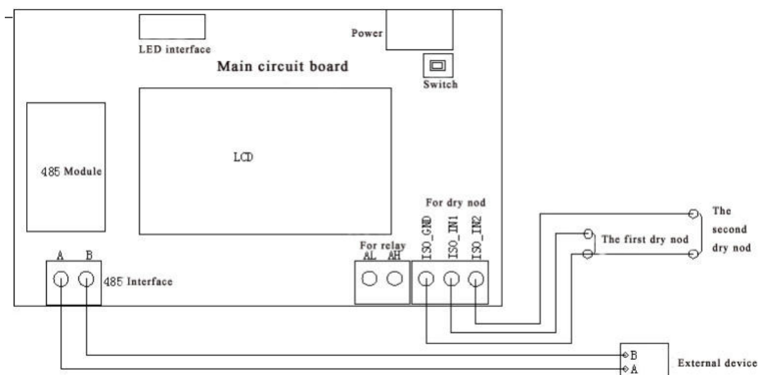
Рисунок 5.2 Схема подключения
